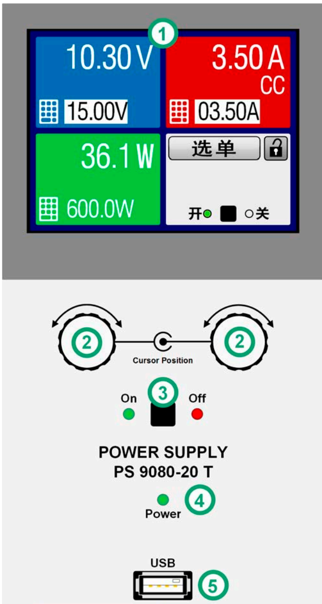
图 6 - 控制面板
